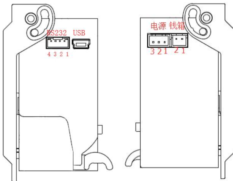
串口通訊 PH02.0mm/4Pin
